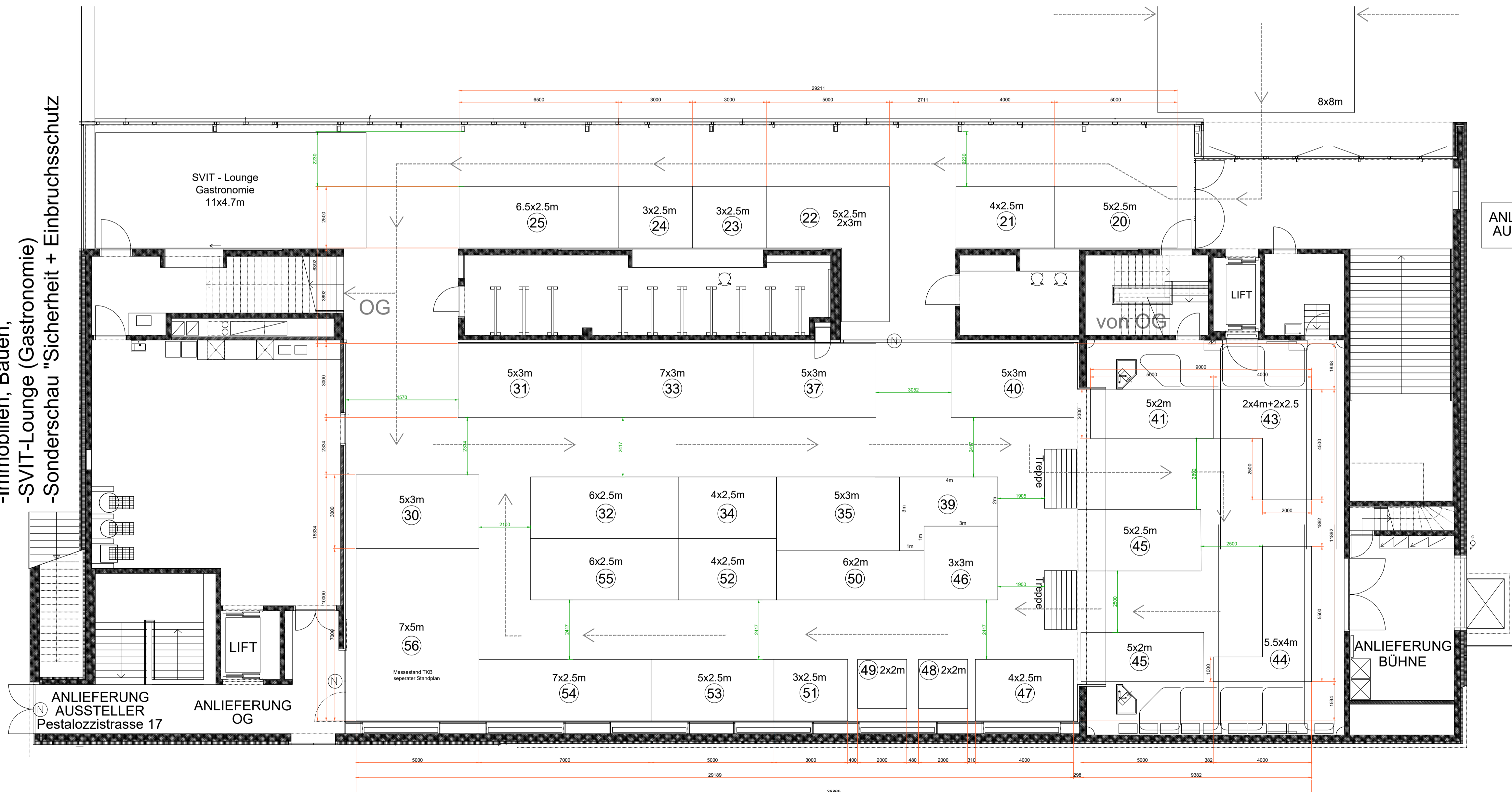
GRUNDRISS OG MST 1:100 - A1
