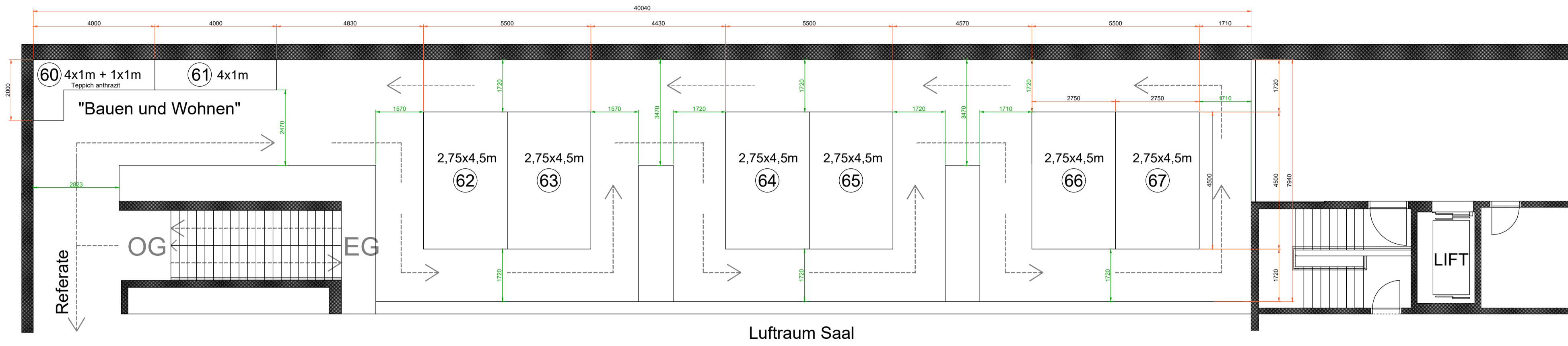
GRUNDRISS OG MST 1:100 - A1
